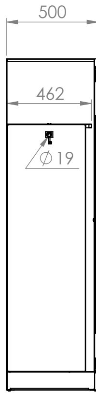
SECTION D-D
