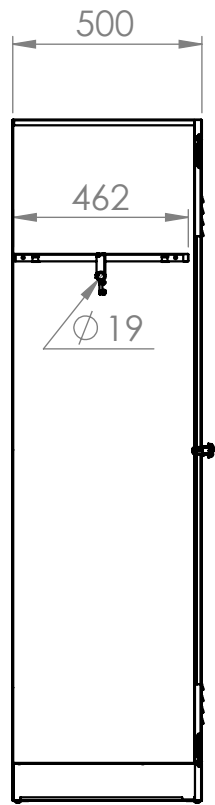
SECTION D-D
